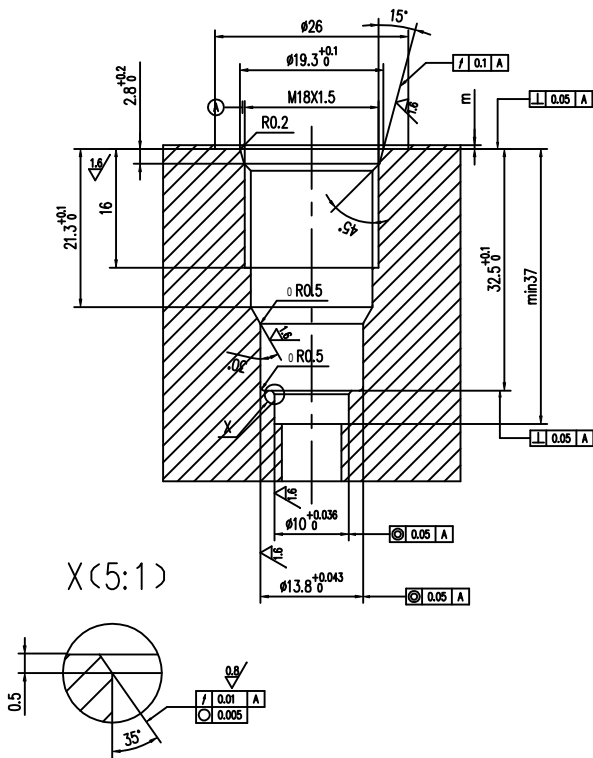
VH002插孔
